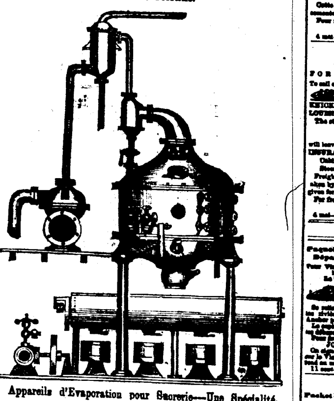
Appareils d'Evaporation pour Saurorie—Une Spécialité
